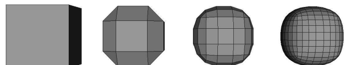
Doo-Sabin
