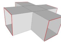
(0) 18 faces
